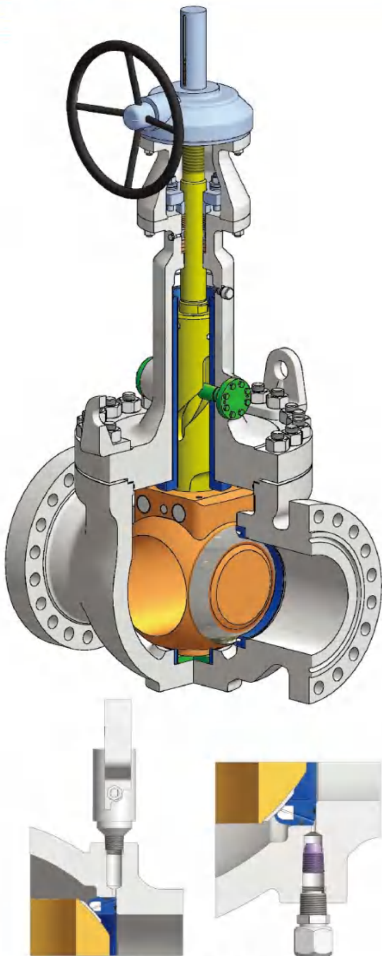
阀座在线检漏及注脂结构说明
