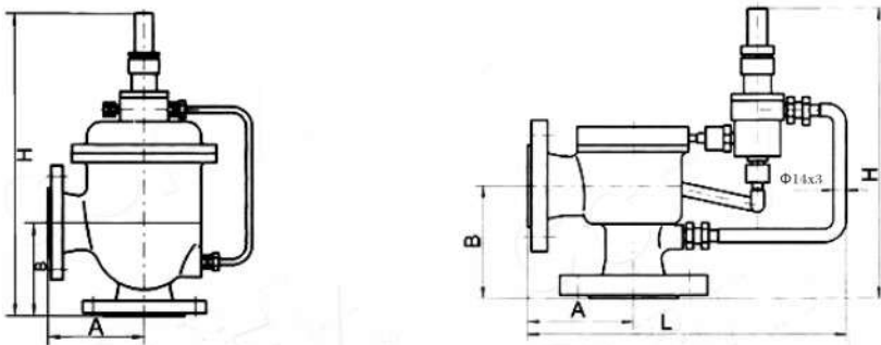
(K)AX46Y F -16C,25,40,64,100主要尺寸表
